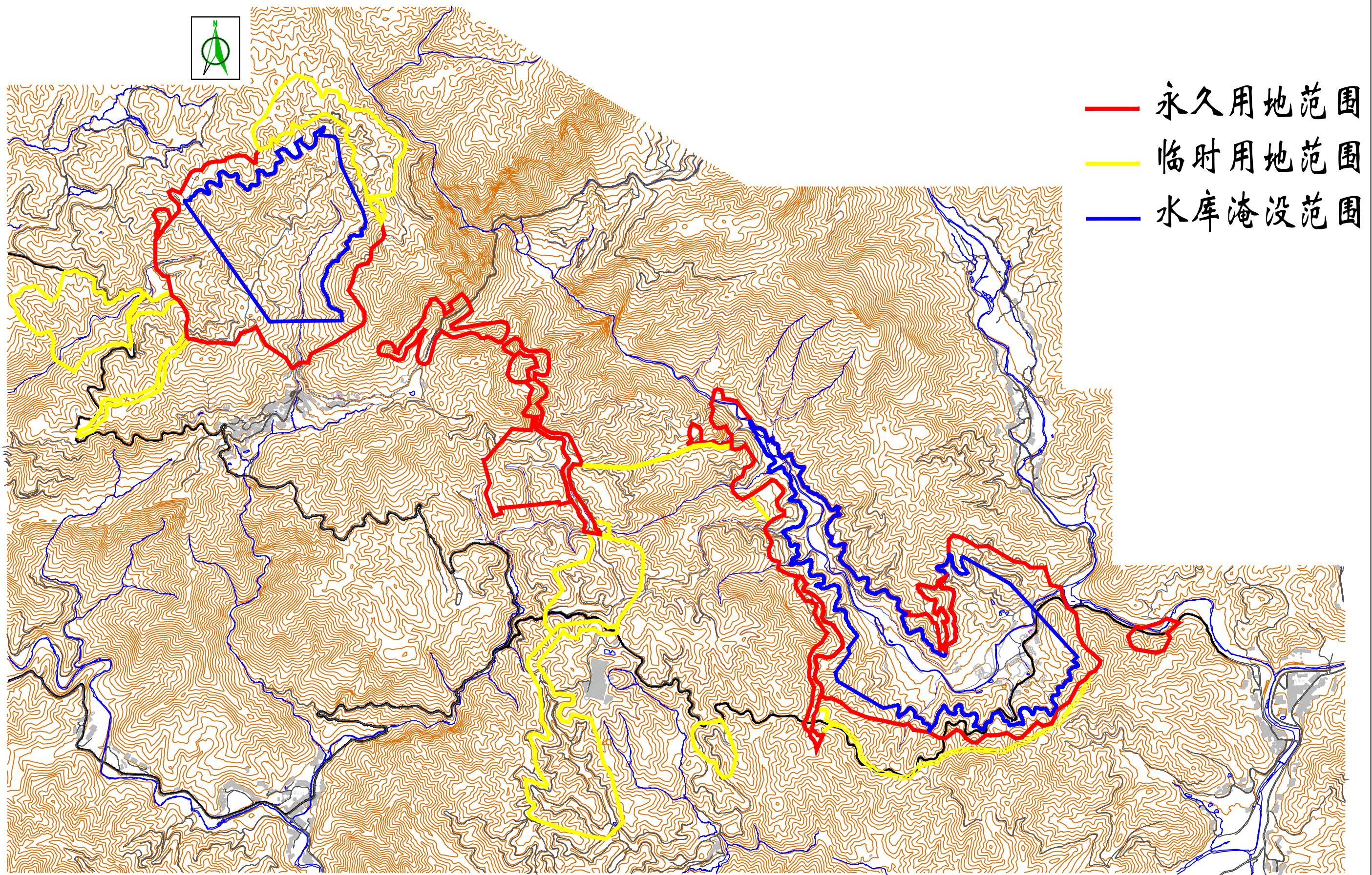
福建省德化抽水蓄能电站建设征地范围示意图
